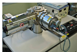
【エッチング】 ECRイオンシャワー装置 (エリオニクス)
