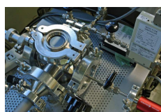
【エッチング】 XeF 2 気相エッチング装置 (自作)
